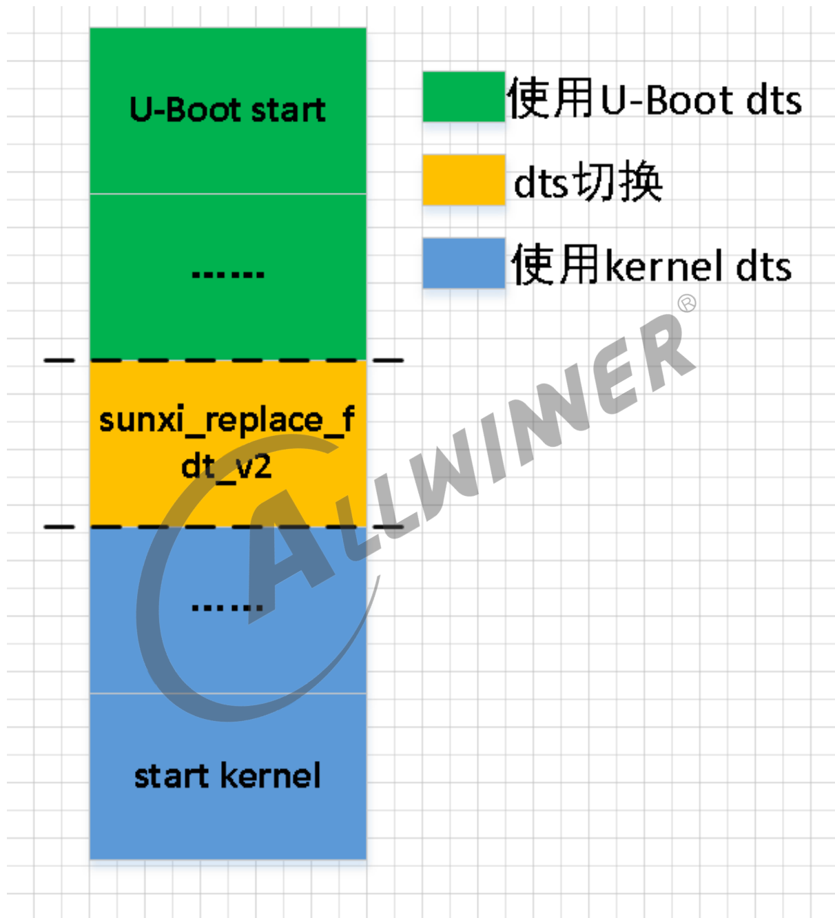
图 4-3: dts 变化图
