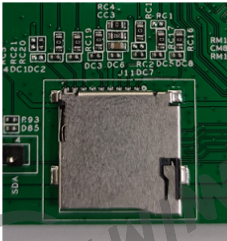
图 5-5: SD 卡槽
