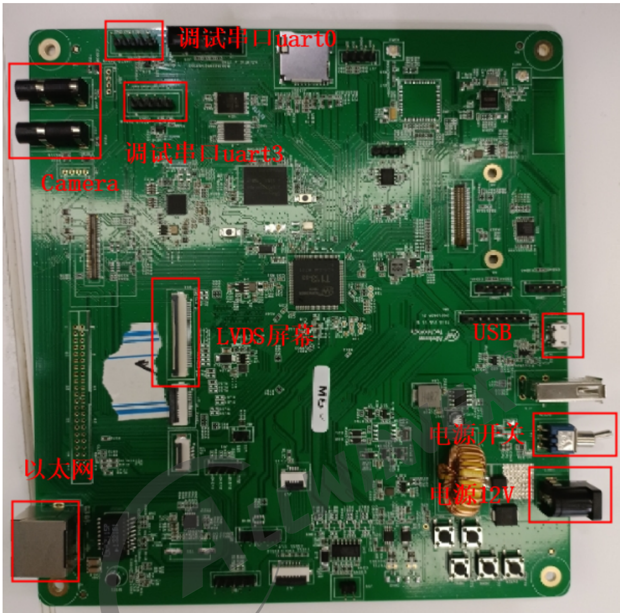
图 3-4: 开发板介绍
